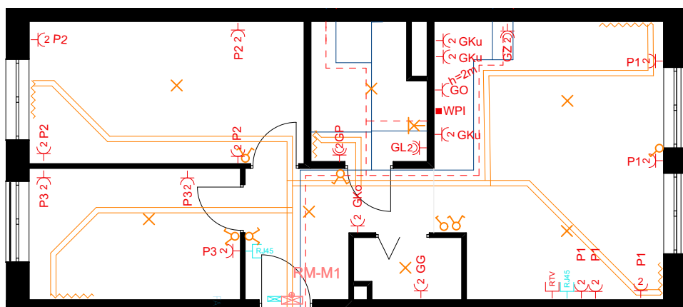
1:100
