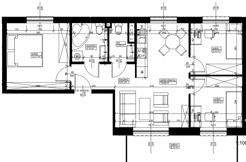
SCHEMAT ZABUDOWY
