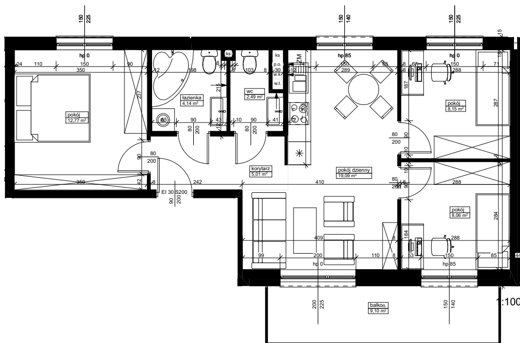
SCHEMAT ZABUDOWY
