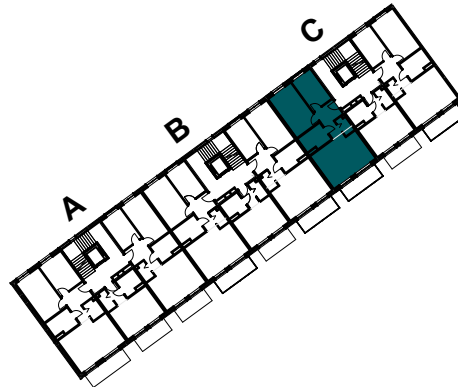
SCHEMAT KONDYGNACJI
