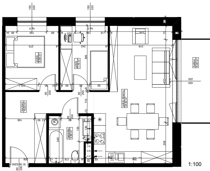
SCHEMAT ZABUDOWY
