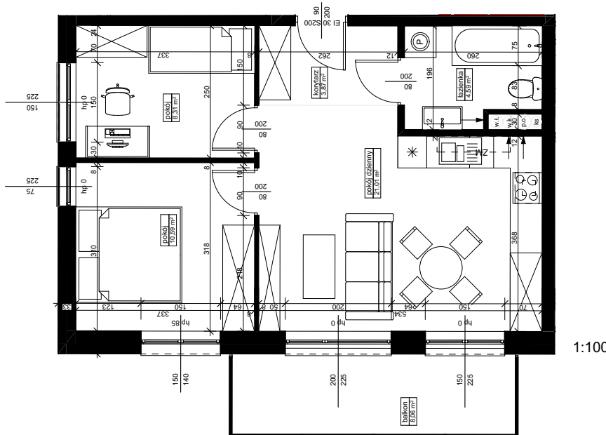
SCHEMAT ZABUDOWY
