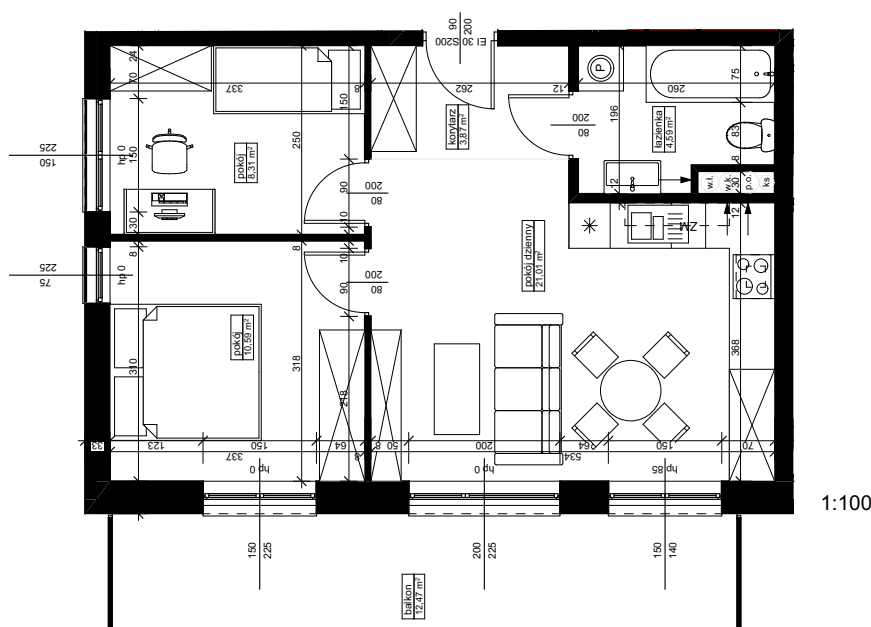
SCHEMAT ZABUDOWY
