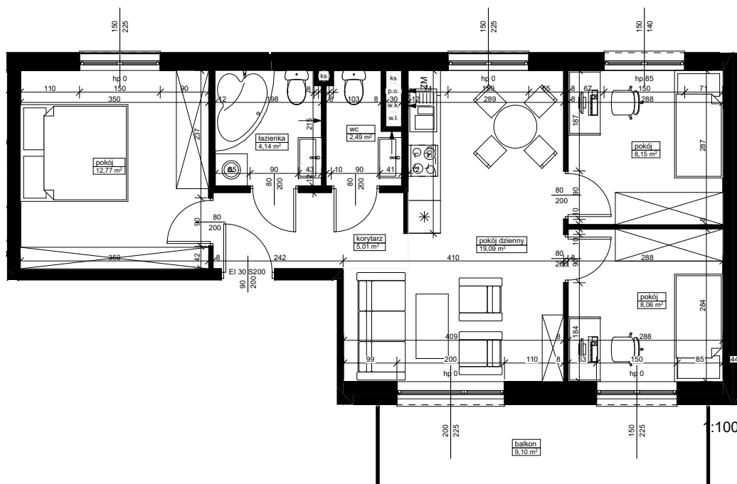
SCHEMAT ZABUDOWY
